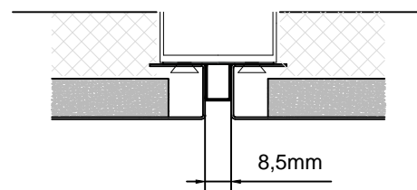
LISTWA OZDOBNA (NP. INOX)
